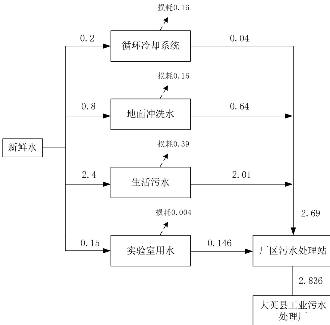
图 3-2 项目水平衡示意图 (m³/d)
