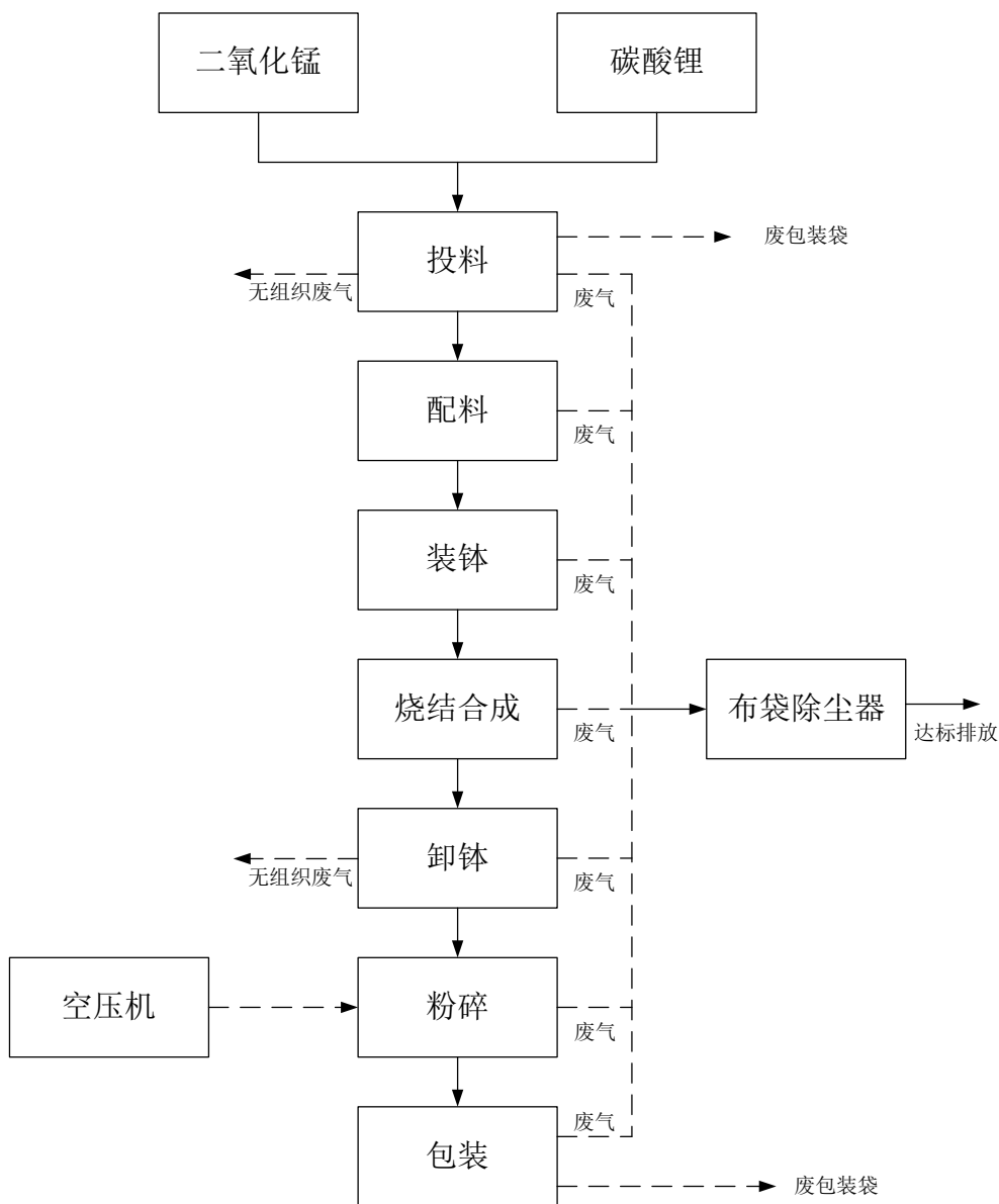
图 3-3 锰酸锂生产工艺流程及产排污环节示意图
