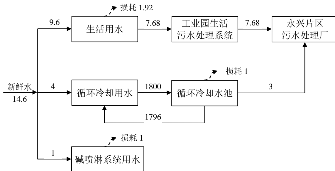
图 3-1 项目水量平衡
